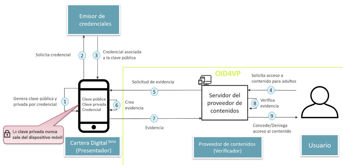
Figura 2. Flujo general: OID4VP
