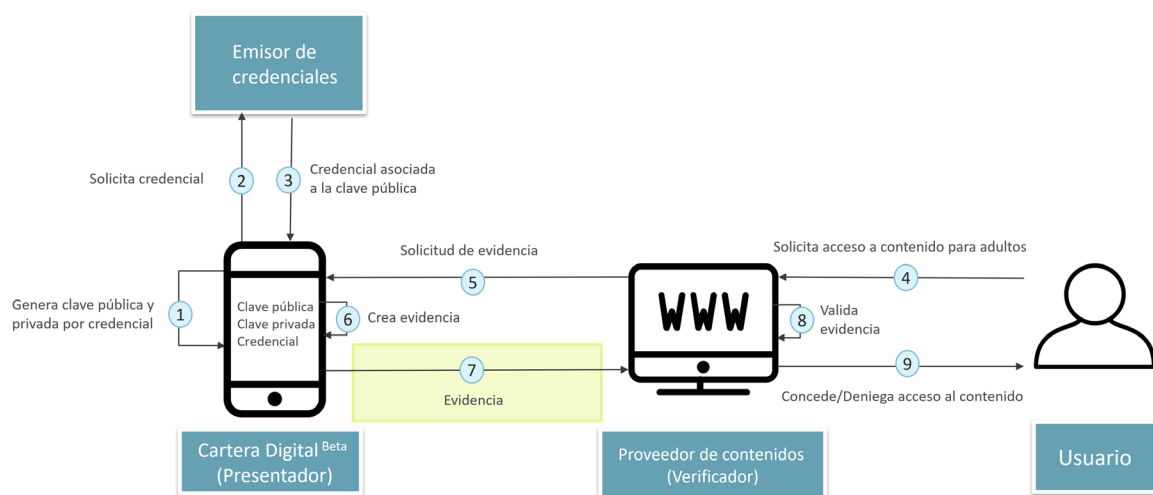
Figura 4. Flujo general: Evidencia
