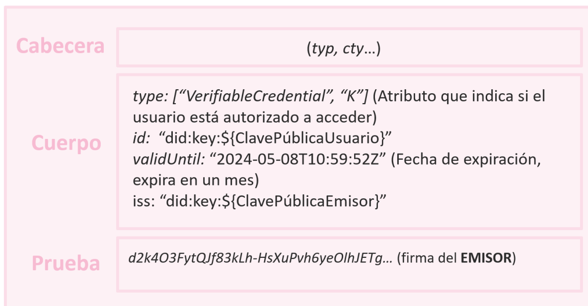
Figura 6. Credencial verificable de tipo K
