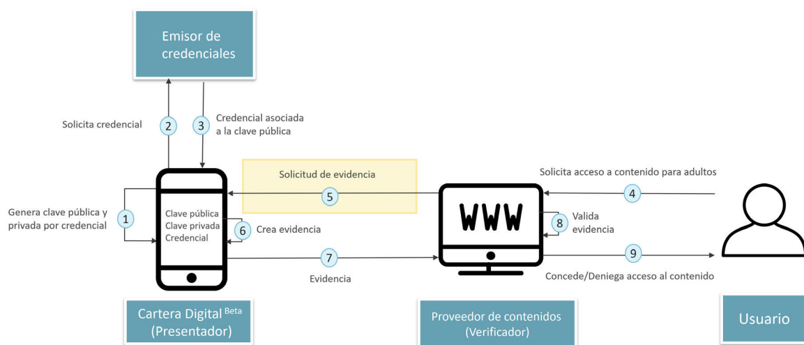
Figura 3. Flujo general: Solicitud de evidencia
