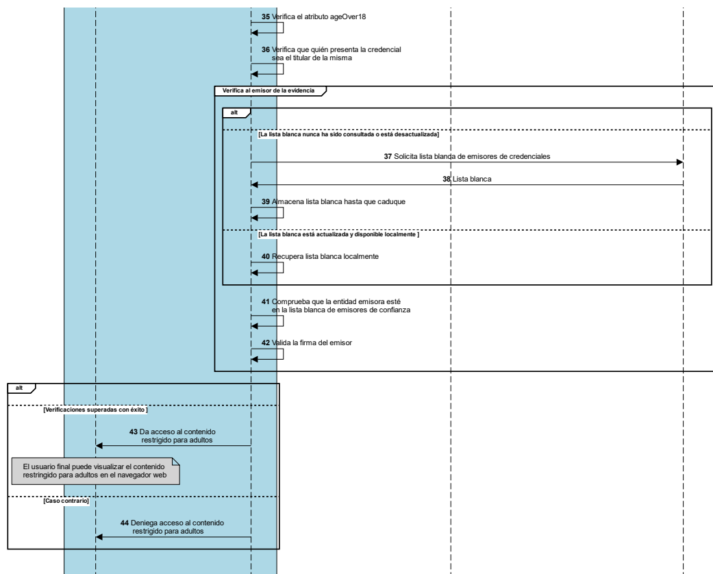
Figura 9. Flujo OID4VP
