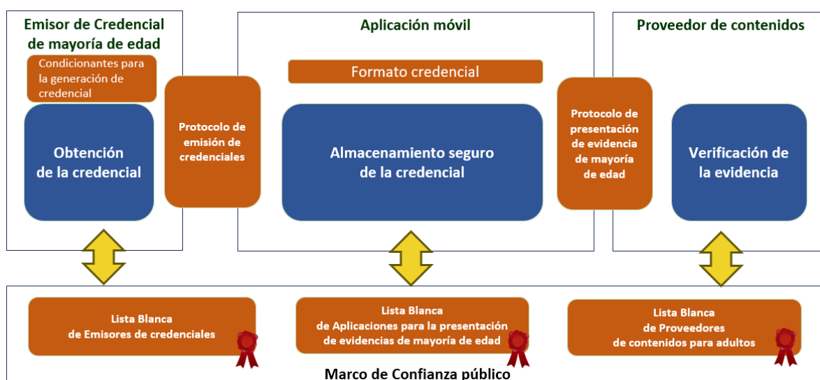
Figura 1. Componentes solución general
